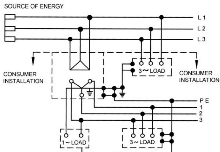
FIG. 16 T-TN-S SYSTEM
